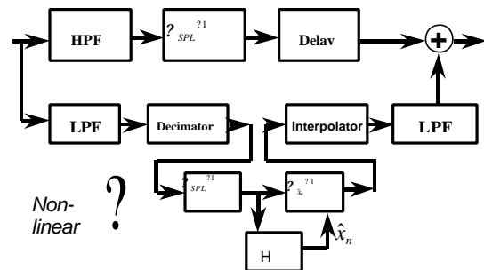
Figure 2 Multirate non linear audio processor.
